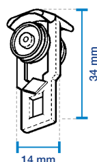
SUSPENDEUR
