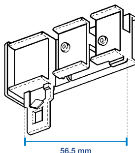
POULIE DE TIRAGE
