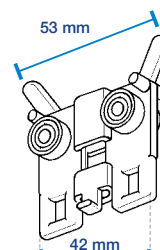
CONDUCTEUR
