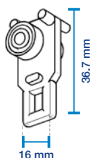
SUSPENDEUR
