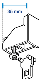
FIXE EMBOUT
