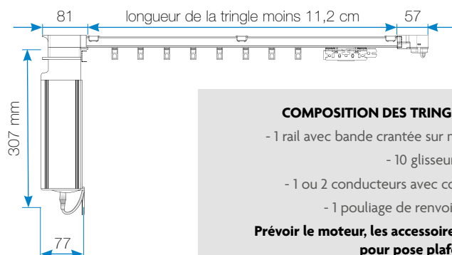
Tringle motorisée SHUTTLE® L (40 W) pour 1 rideau
