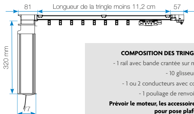
Tringle motorisée SHUTTLE® iOn (30 W) pour 1 rideau
