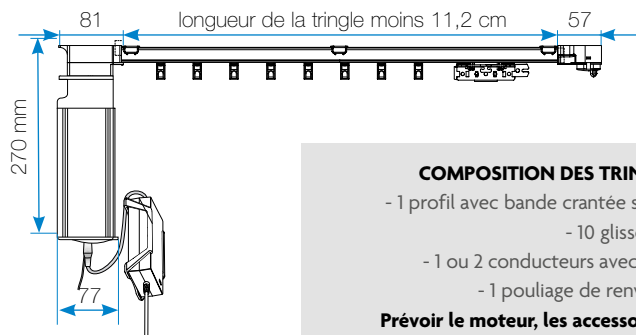
Tringle motorisée SHUTTLE® M (65W) pour 1 rideau
